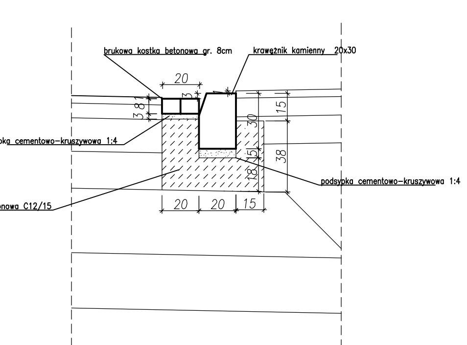
Szczegół G węznik drogowy zatopiony ze ściekiem przykrawężnikowym
