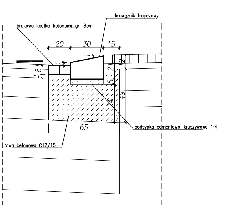
Szczegół H węznik trapezowy ze ściekiem przykrawężnikowym
