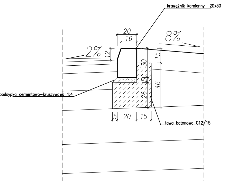
Szczegół F krawężnik drogowy bez ścieku zykrawężnikowego na krawędzi jezdni
