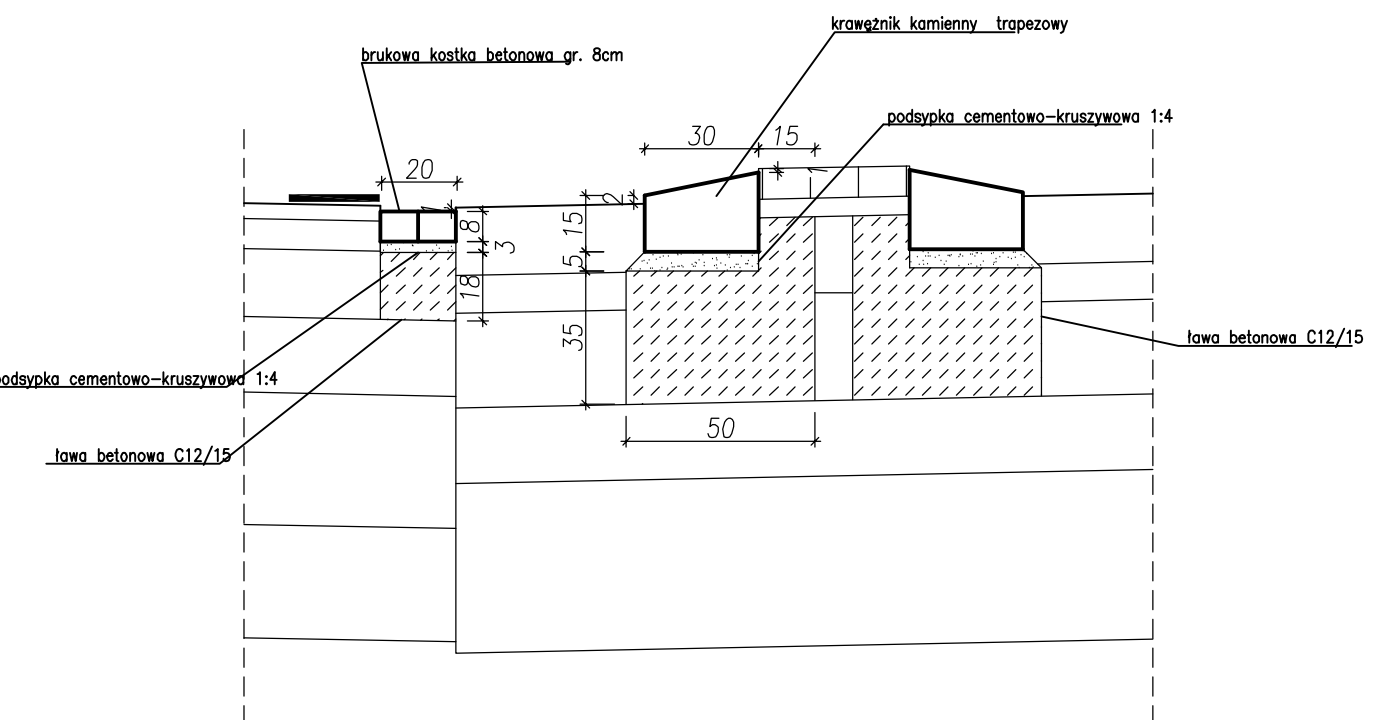
Szczegół G węznik drogowy zatopiony ze ściekiem przykrawężnikowym
