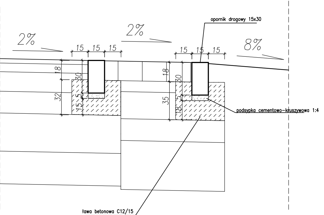
Szczegół C pornik drogowy z zabrukowaniem na skrzyżowaniach
