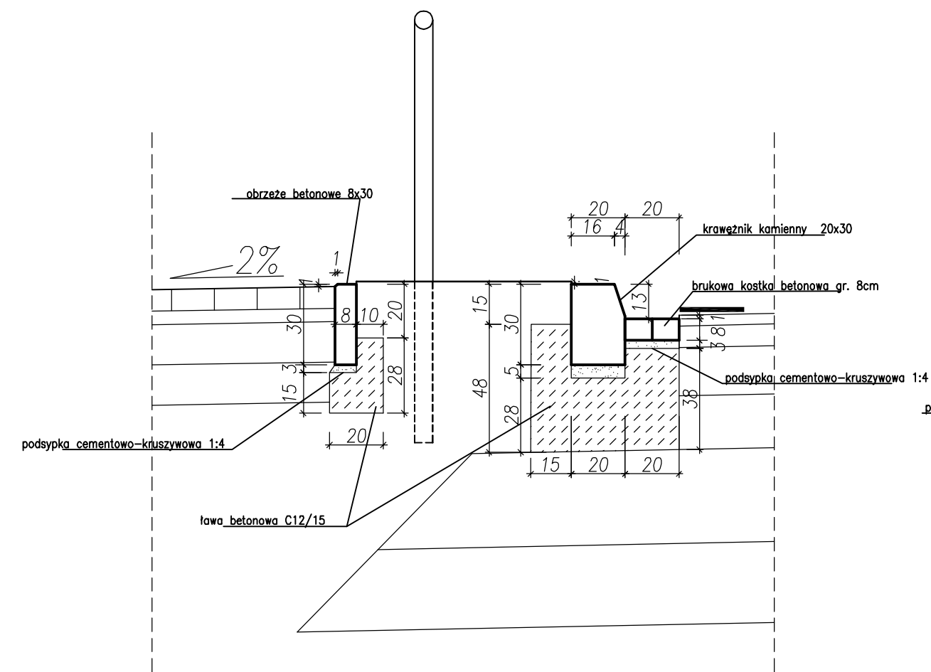
Szczegóły A prawy drogowy ze ściekiem przykrawężnikowym z kostki brukowej grubości 8 cm obrzeże betonowe przy chodniku
