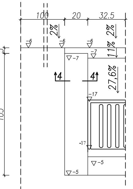
Szczegół N budowa od strony zakończenia cieku trójkątnego studzienką widok z góry
