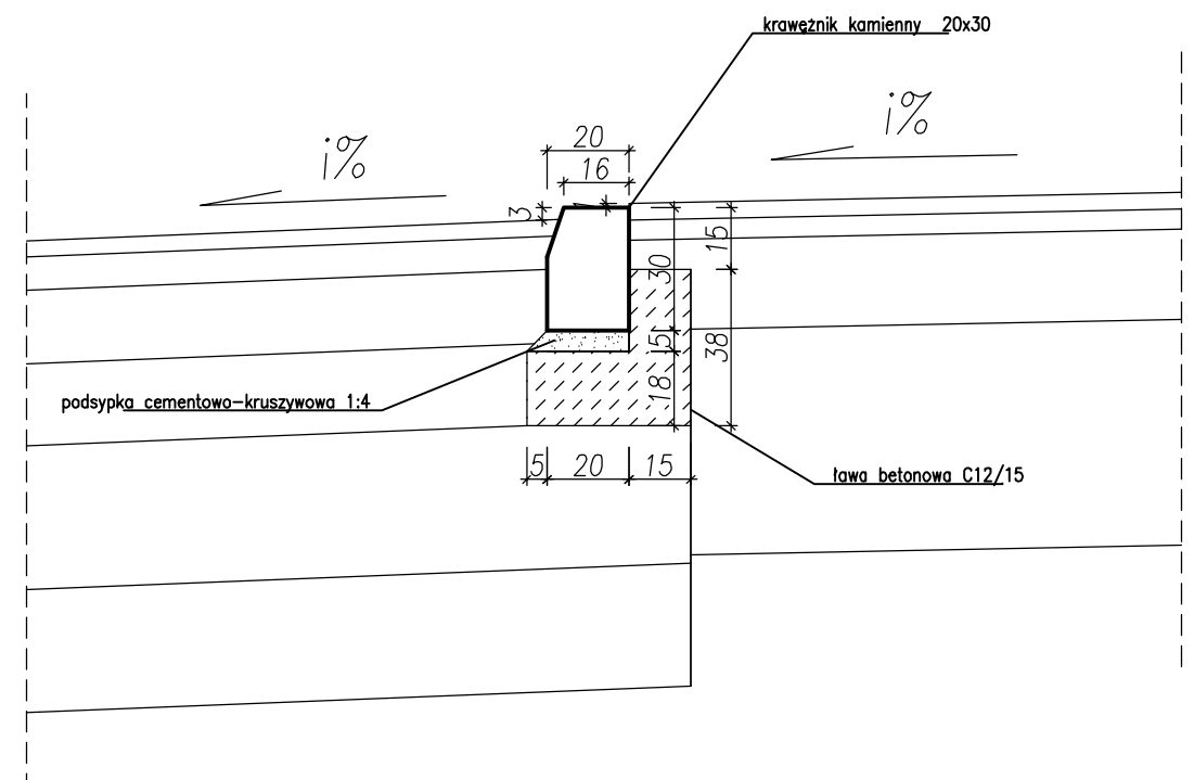
Szczegół D Zawężnik drogowy zatopiony na zjazdach publicznych/indywidualnych
