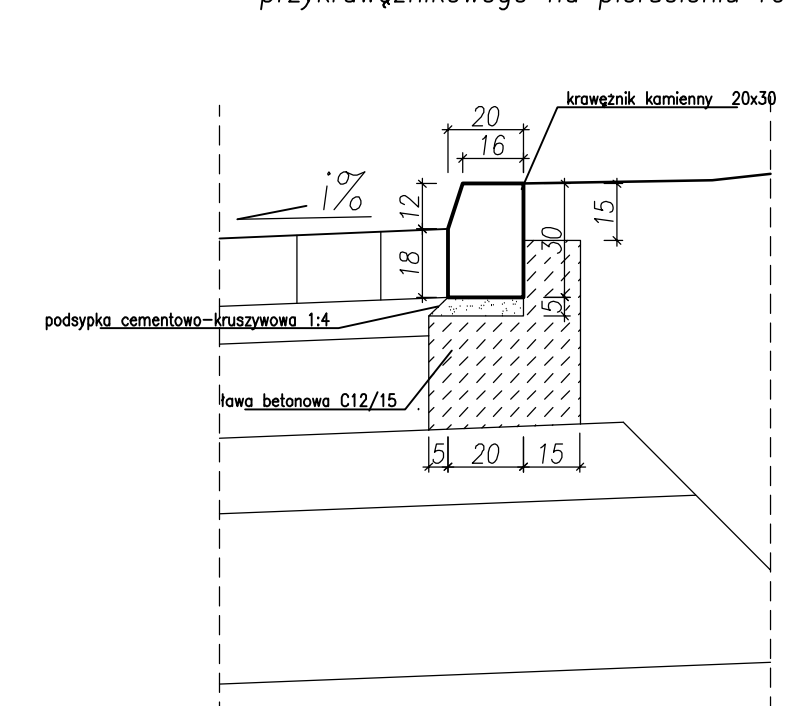
Szczegół E krawężnik drogowy bez ścieku rzykrawężnikowego na pierścieniu ronda
