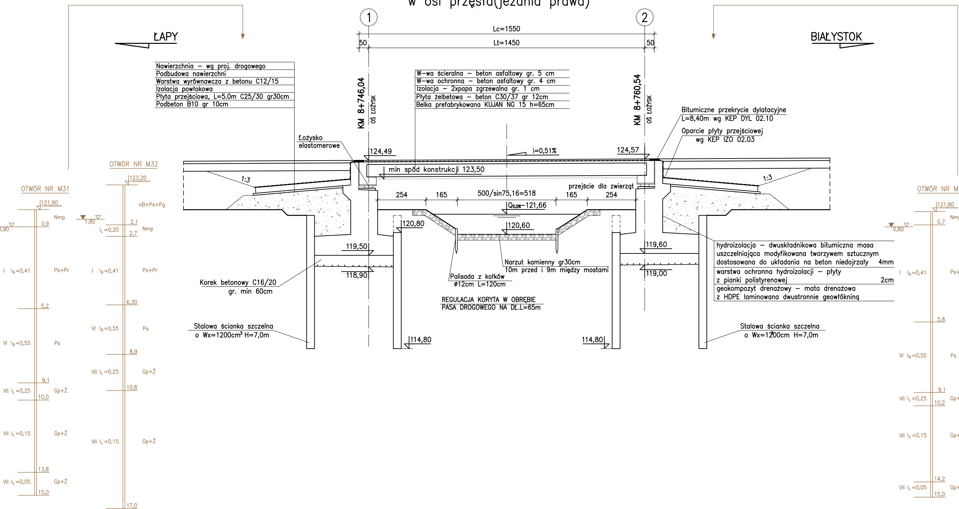
PRZEKRÓJ PODŁUŻNY 1:100 w osi przęsła (jezdnia prawa)
