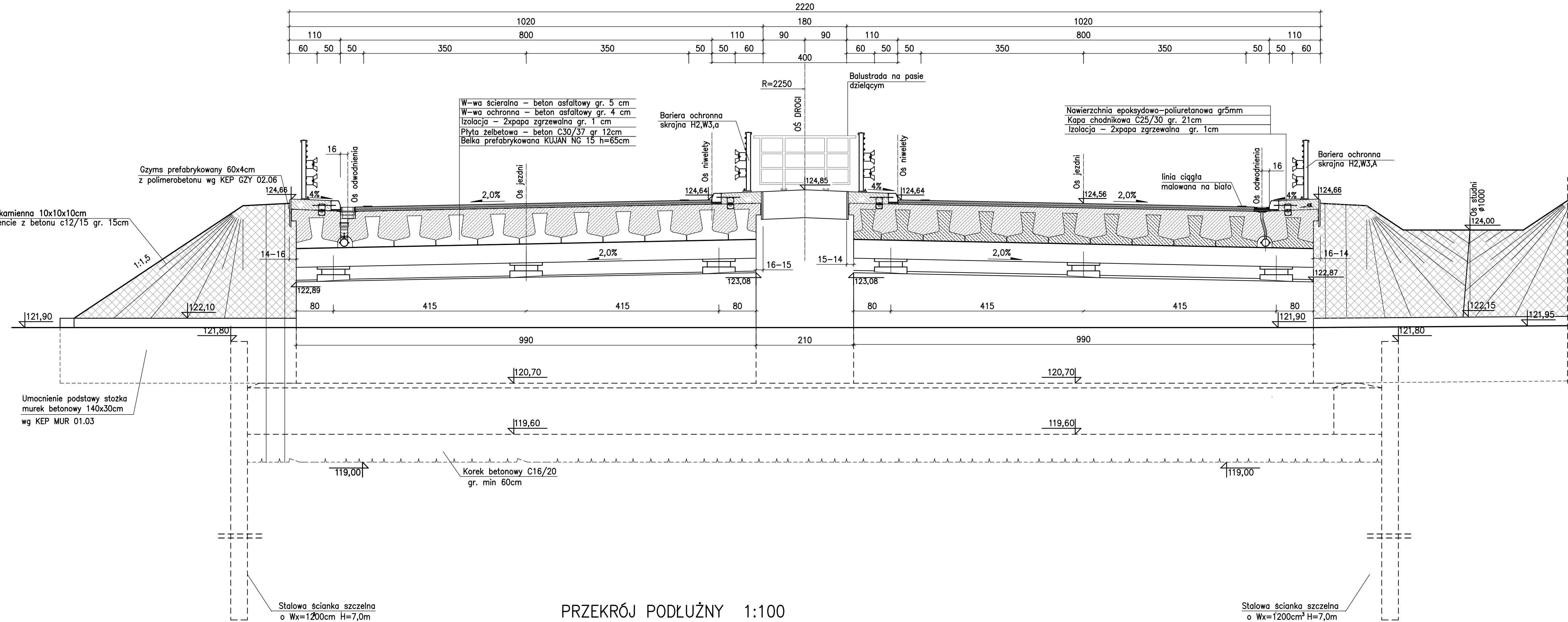
PRZEKRÓJ PODŁUŻNY 1:100 w osi przęsła (jezdnia prawa)
