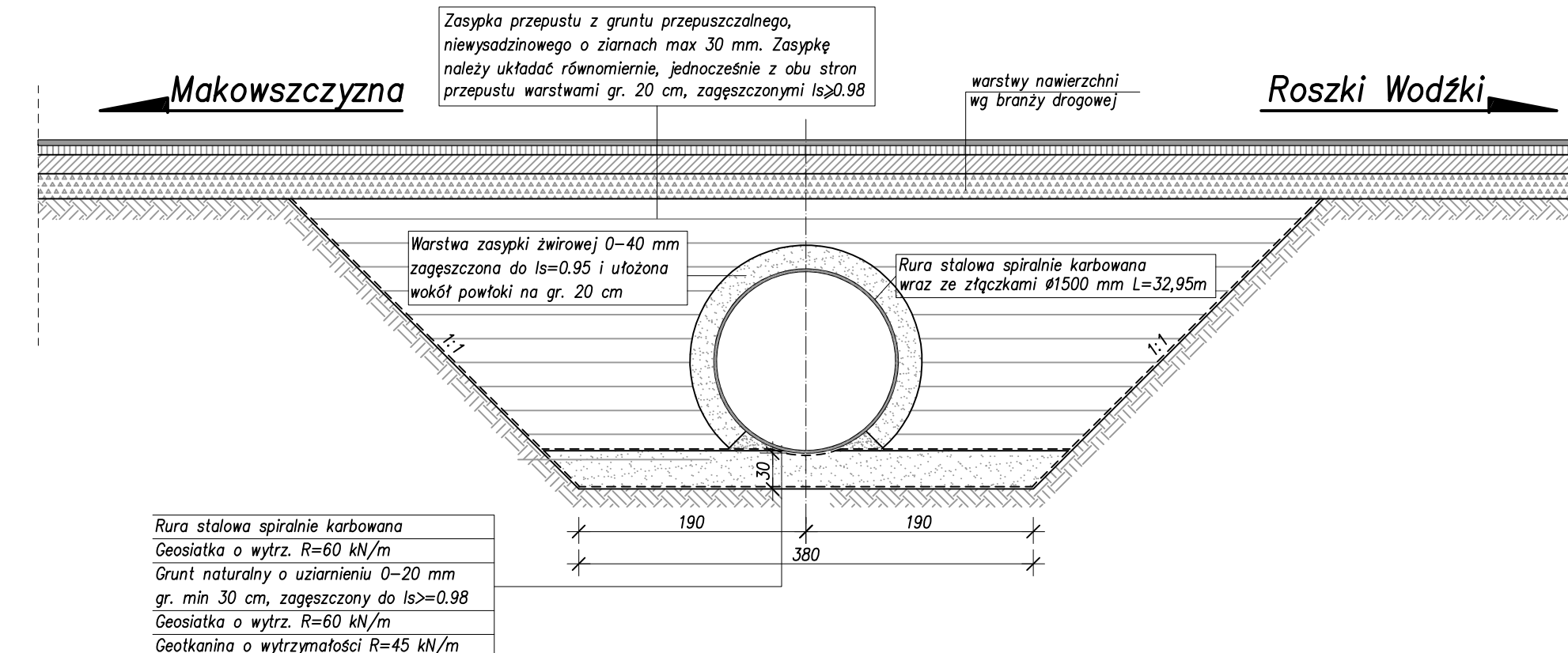
PRZEKRÓJ POPRZECZNY W OSI JEZDNI (B-B) Skala 1:50
